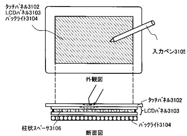
(b) 携帯情報端末機器(ペン入力式タッチパネル)の外観図および断面図
