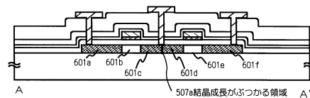
(B) A-A' 断面図
