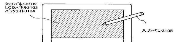
(a) 携帯情報端末機器(光学式タッチパネル)の外観図および断面図
