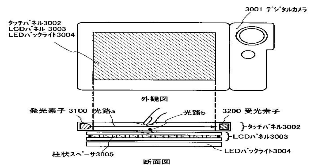
(a) 携帯情報端末機器(光学式タッチパネル)の外観図および断面図
