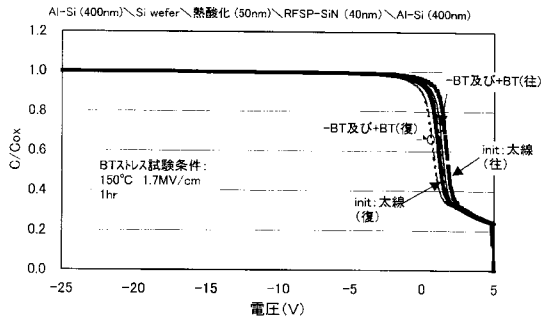
(A) Li拡散源がない場合のMOS構造におけるC-V特性
