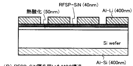
(B) RFSP-SiN膜を用いたMOS構造
