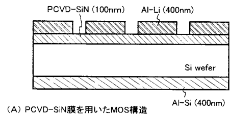
(A) PCVD-SiN膜を用いたMOS構造
