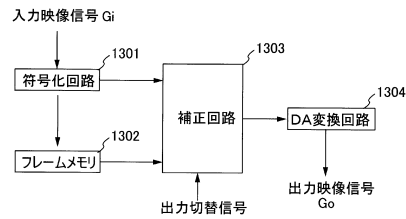
(B) オーバードライブ回路 (アナログ)
