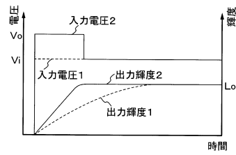
(B) オーバードライブ回路 (アナログ)
