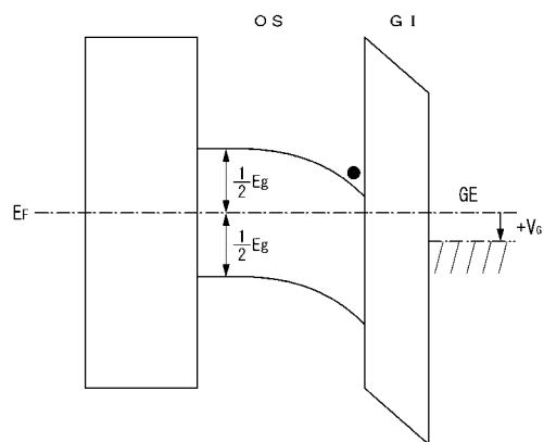
(A) B-B' 断面エネルギーバンド図 (+V g )
