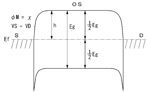
(A) A-A' 断面エネルギーバンド図
