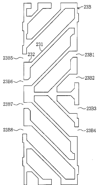
図23中のコモン電極のパターン図
