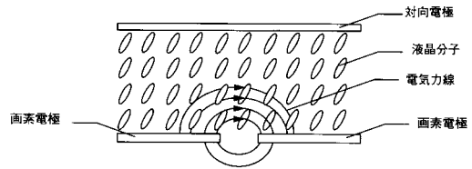
(B) (電圧印加直後の状態時での(液晶分子が反応する前))画素間に発生する電気力線の状態モデル図(断面図)
