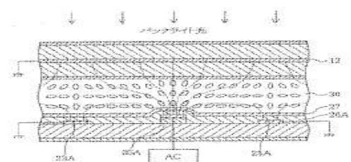
図16の液晶画面の電圧印加状態を示す概略断面図
