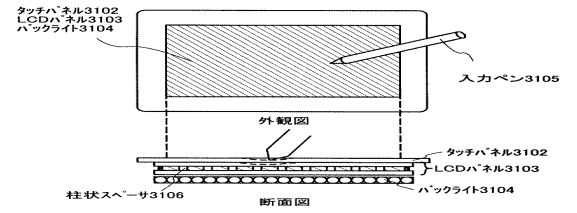
(b) 携帯情報端末機器(ペン入力式タッチパネル)の外観図および断面図
