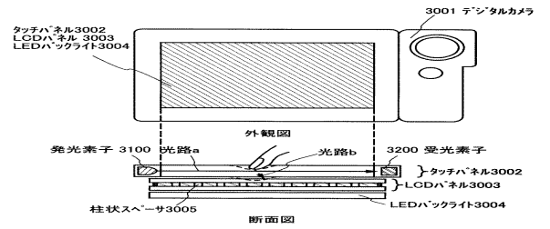
(a) 携帯情報端末機器(光学式タッチパネル)の外観図および断面図
