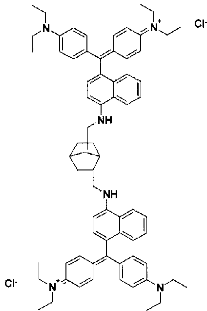
化学式 (2)
