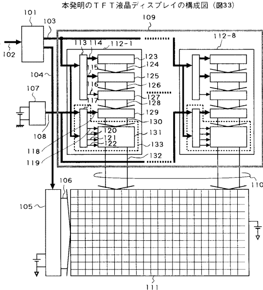
本発明のTFT液晶ディスプレイの構成図 (図33)
