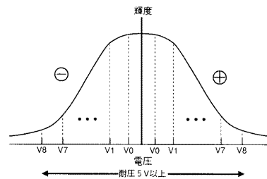
T F T 液晶の電圧輝度特性図 (図54)
