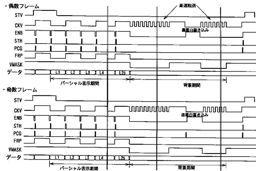
パージアル表示時のタイミングチャート（駆動方法3及び4）
