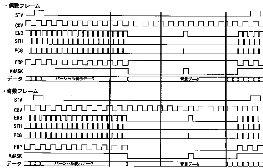
パージアル表示時のタイミングチャート（駆動方法3）
