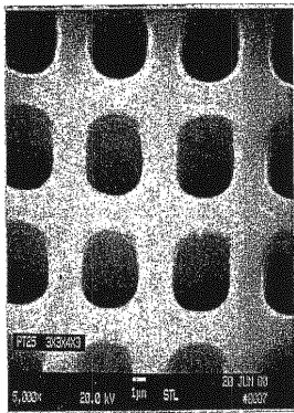
FIG. 4a マイクロカップのSEM写真 4.3 x 4.3 x 4.4 x 2.4 \mu\text{m} (5000x) (L x W x D x 壁) 開口面積 41%
