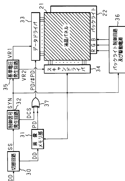
実施の形態１に係る本発明の液晶表示装置の構成を示すブロック図
