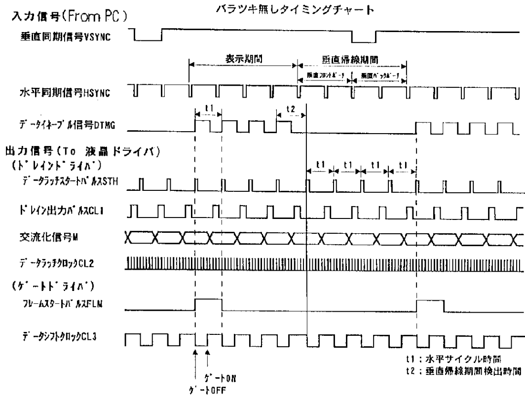
液晶ドライバの入カシーケンス (例)
