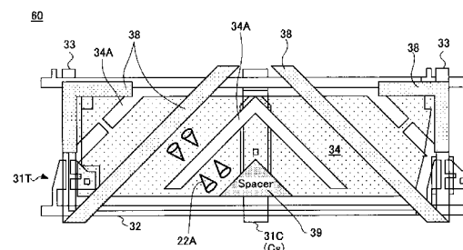
本発明第3実施例による液晶表示装置における画素の構成を示す図
