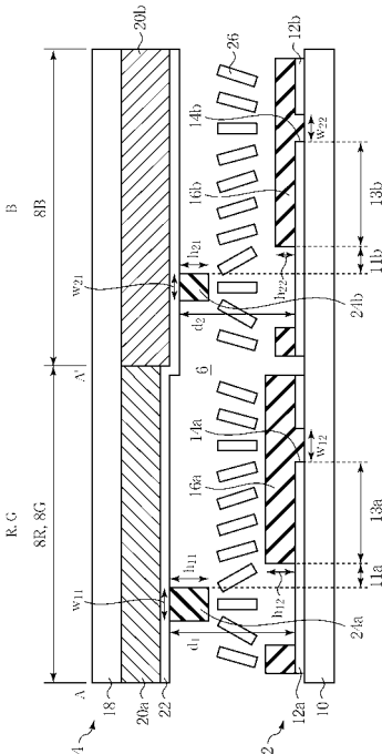
本発明の第1実施形態による液晶表示装置を示す断面図
