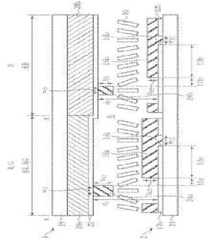
本発明の第2実施形態による液晶表示装置を示す断面図
