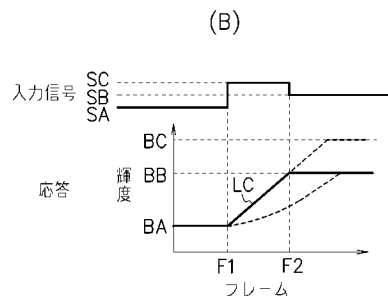
第1の問題点を説明するための図
