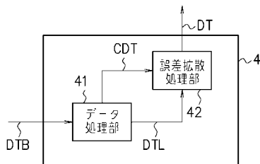
第 2 の実施形態の構成例
