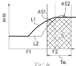
第 3 の実施形態
