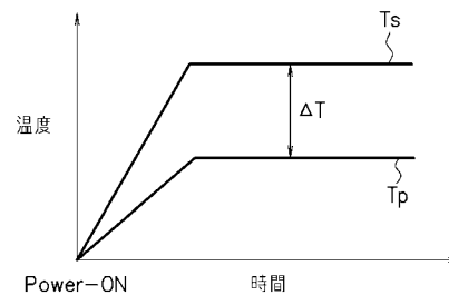
第4の問題点を説明するための図
