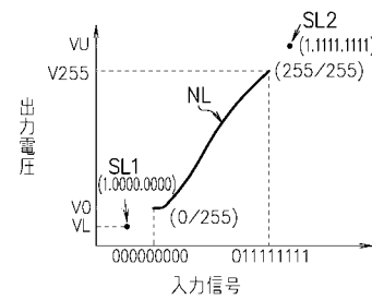
第 1 の実施形態の出力レベルの他の例
