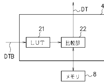
第 1 の実施形態の構成例
