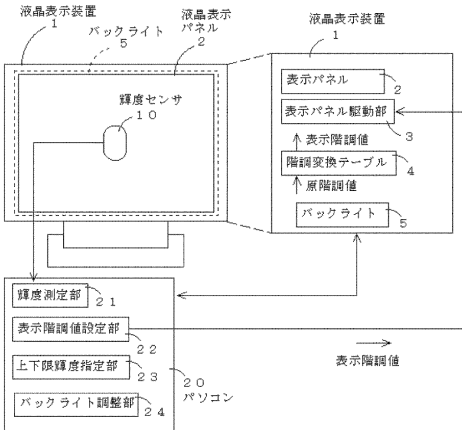
階調調整装置 100
