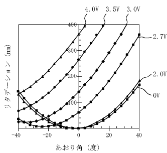
(a) y z 面内リタデーション
