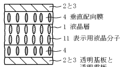
(c) x z 面断面図
