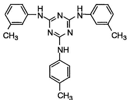
I-(6)
