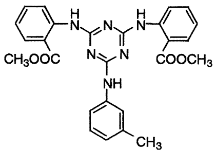
I-(15)
