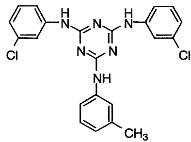
I-(46)
