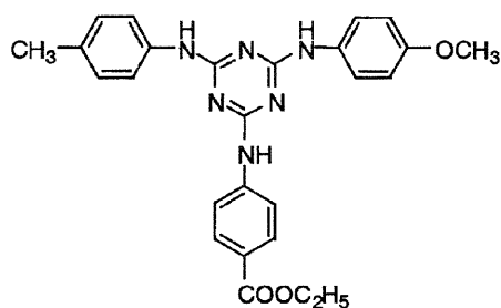
IV-(9)
