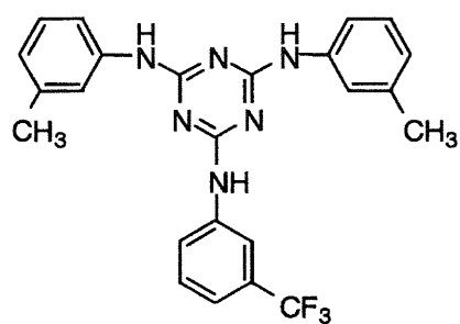
I-(20)
