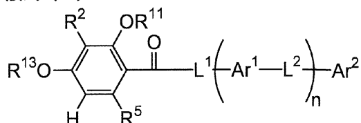
一般式 (IV)
