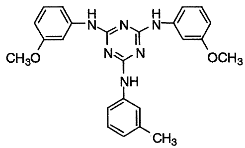
I-(40)
