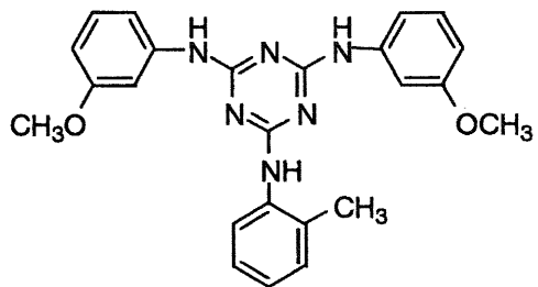
I-(37)
