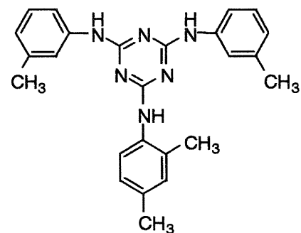
I-(8)
