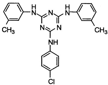
I-(13)
