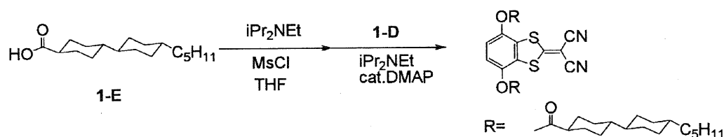
例示化合物(1)
