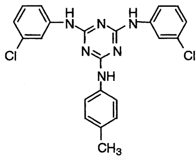
I-(47)
