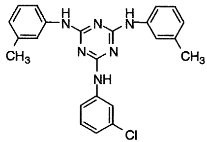
I-(14)
