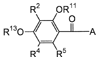
構造体 A
