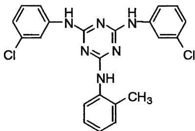
I-(43)
