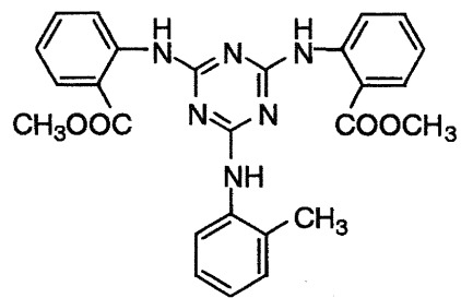
I-(16)
