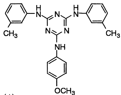
I-(4)
