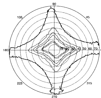
比較例1の等コントラスト曲線
