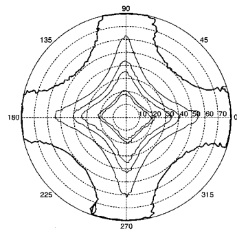
実施例1の等コントラスト曲線
