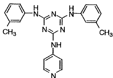
I-(36)
