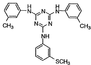
I - (31)
