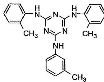
I-(48)
