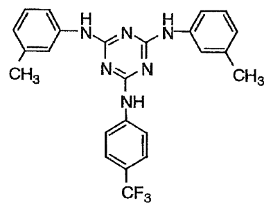
I - (32)
