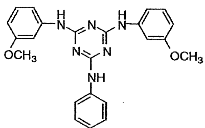
I-(36)
