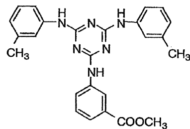
I - (31)
