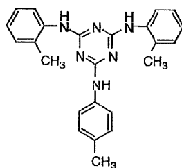
I-(49)
