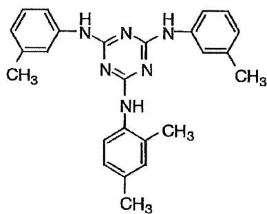
I-(8)
