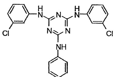
I-(47)
