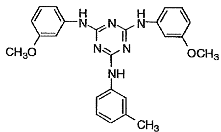
I-(40)
