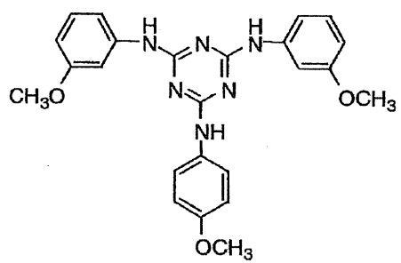
I-(40)
