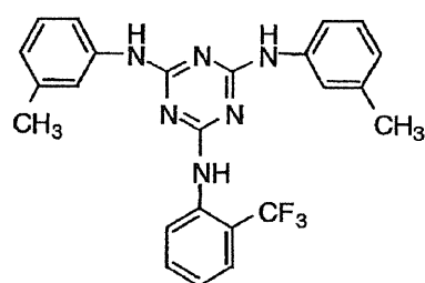
I-(23)
