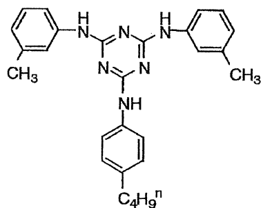
I - (28)
