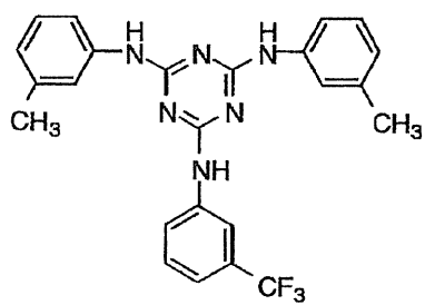
I-(20)
