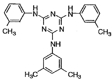
I-(22)
