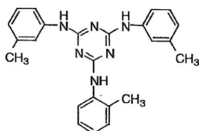
I-(8)
