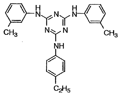
I - (29)
