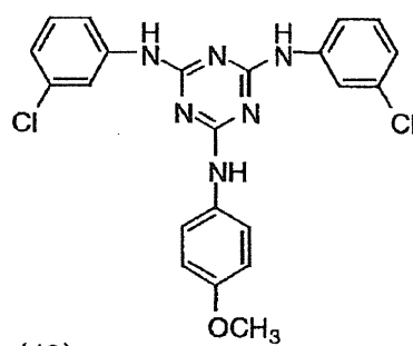
I-(48)
