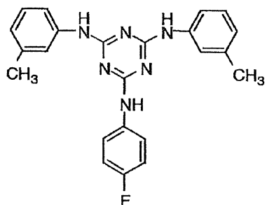
I - (30)
