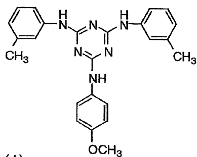
I-(4)
