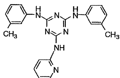
I-(17)
