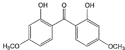
紫外線吸収剤（UV-1）
