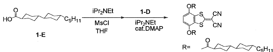
例示化合物(1)
