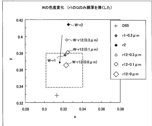
図12の半透過型液晶表示装置全体の反射光の白色度変化を示す別の図
