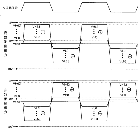
液晶交流出力電圧のタイミング図（図41）
