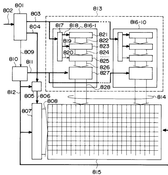
従来の TFT 液晶ディスプレイの構成図 (図 7 3)
