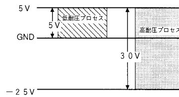
プロセス電圧(図70)
