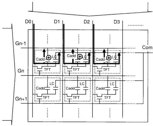
画素部電流方向の説明図（図75）
