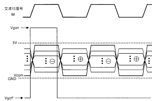
従来技術の液晶基準電圧の交流タイミング図 (図74)
