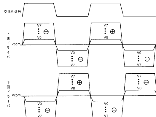
従来技術の液晶基準電圧の交流タイミング図 (図71)
