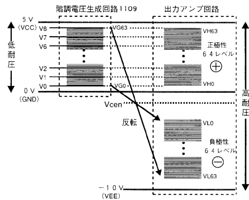
階調電圧反転図 (図40)
