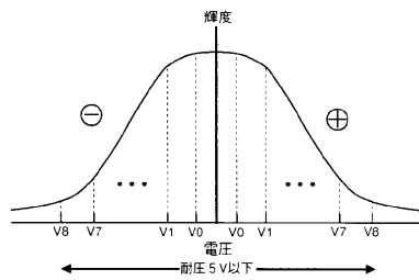
TFT液晶の電圧輝度特性図（図59）
