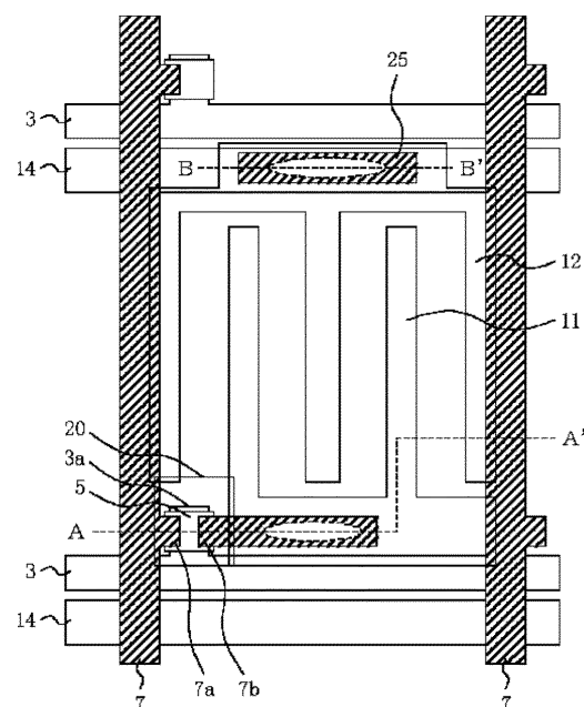
3: 走査線, 7: 信号線, 7a: ソース電極 7b: ドレイン電極, 11: 画素電極, 12: COM電極 14: 共通電極線, 25: 導通部
