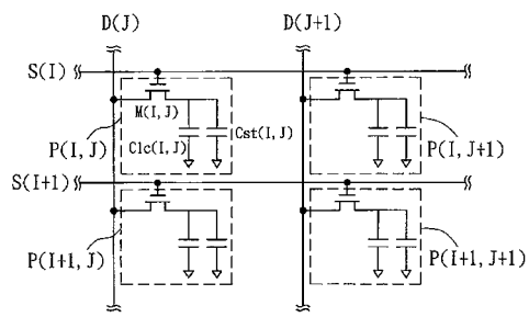
図 1 (従来技術)
