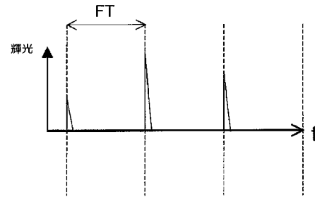
図 3 (従来技術)
