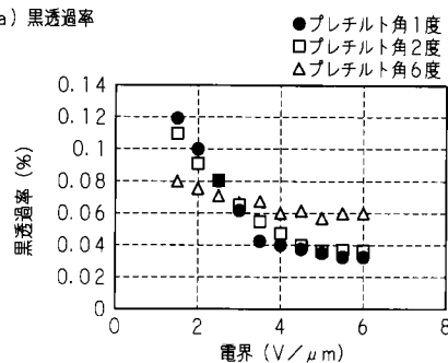
配向処理時の電界と黒透過率／コントラスト比との相関を示すグラフ
