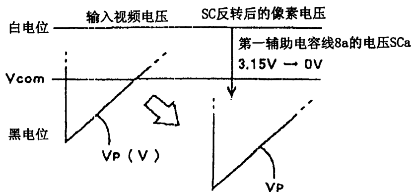
(a) 像素电压 V_p (第一像素GS1)
