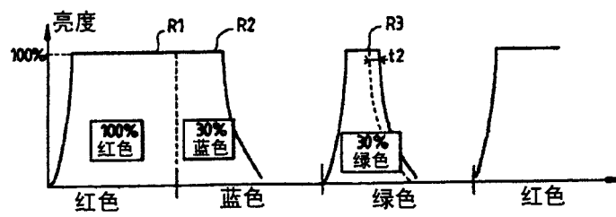
图 4a
