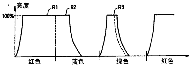
图 5a
