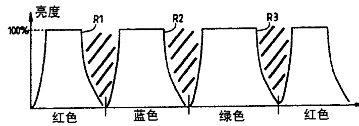
图 3b
