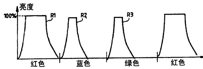
图 3b
