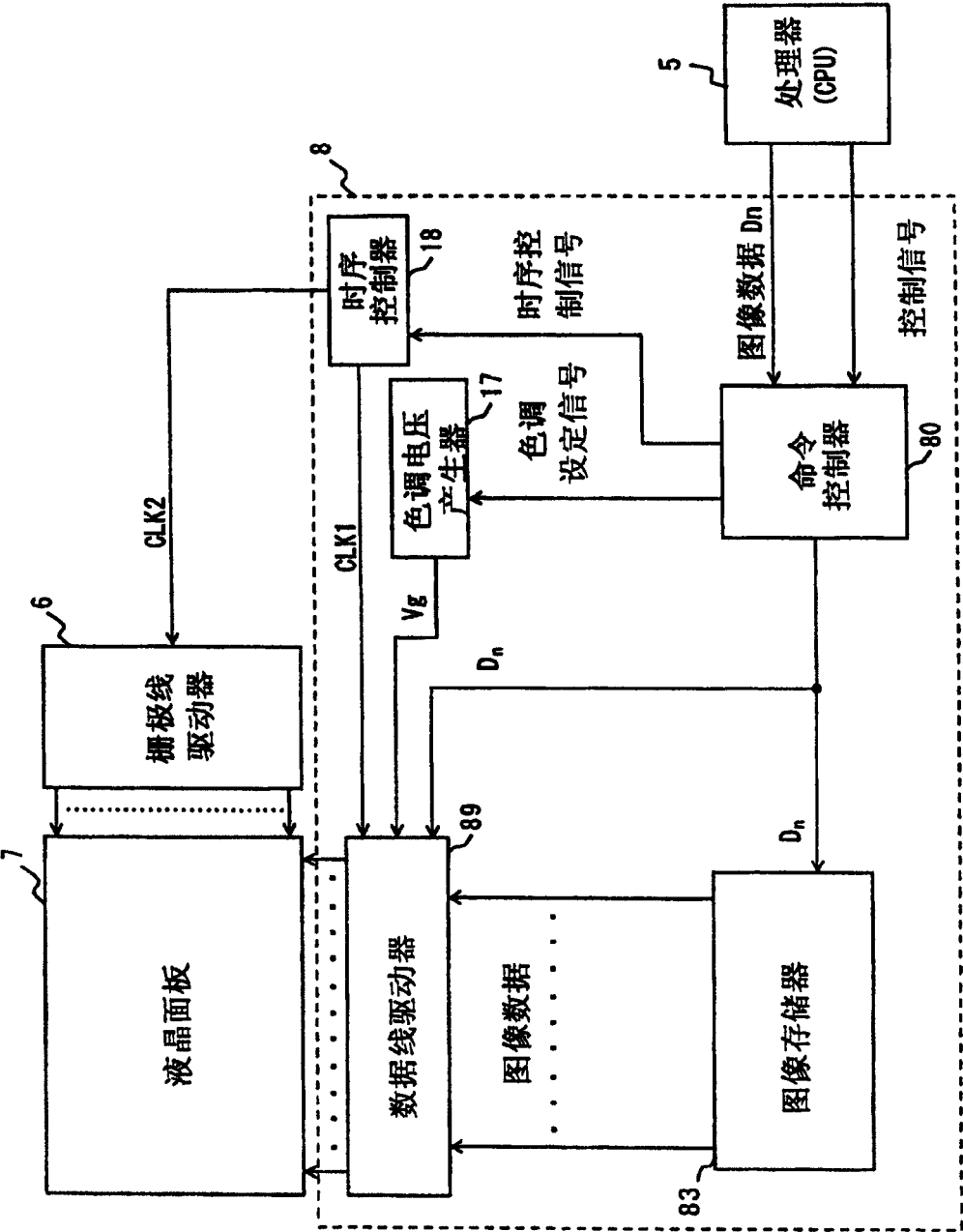
图14 现有技术
