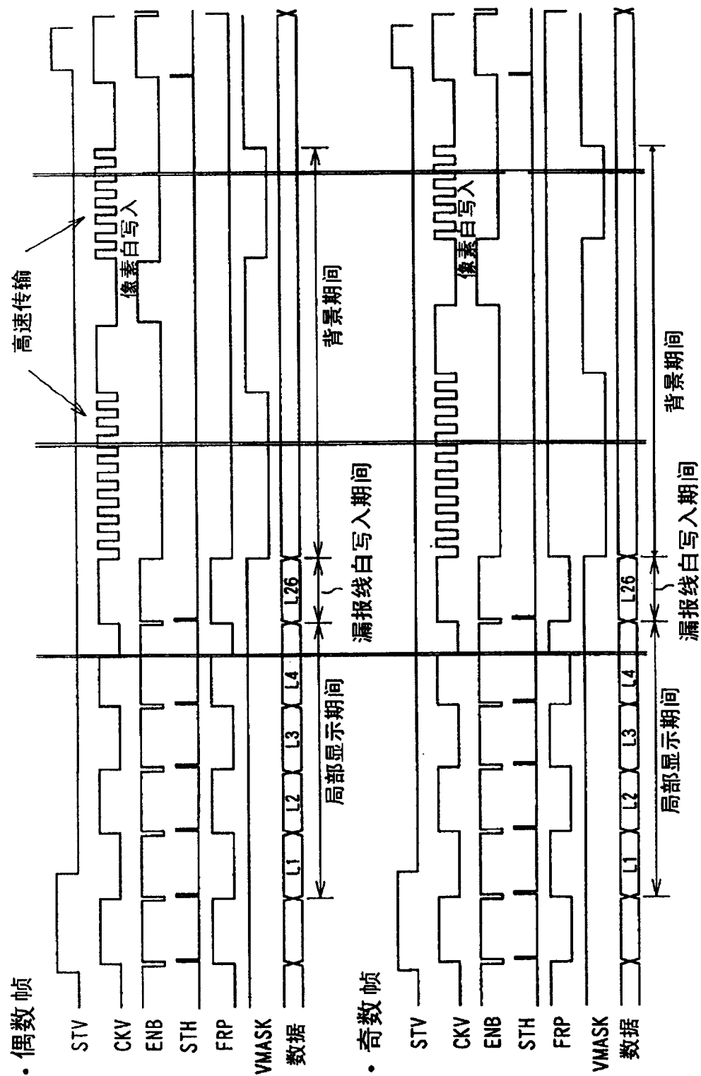
局部显示时的时序图(驱动方法2以及4)
