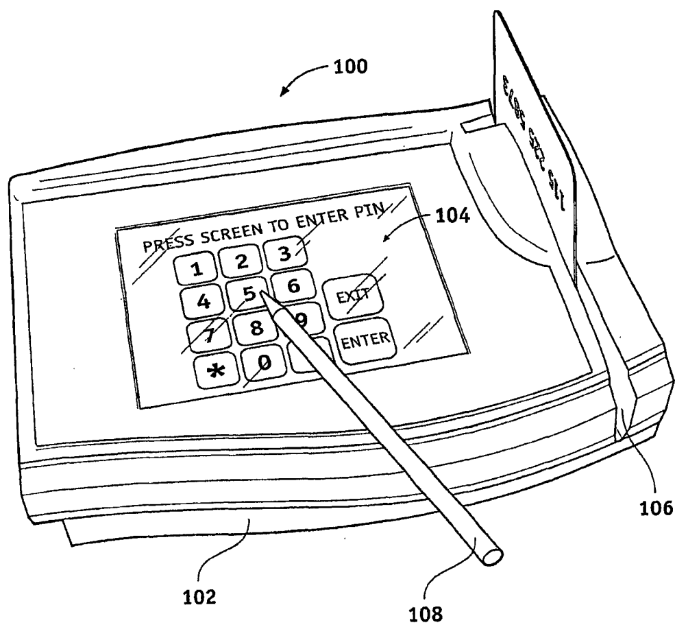
图1 (现有技术)
