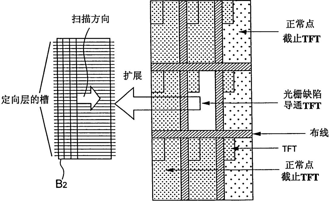
从TFT侧（0度方向）消除定向层的槽
