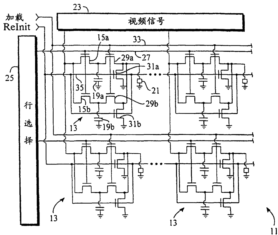
图 4(现有技术)
