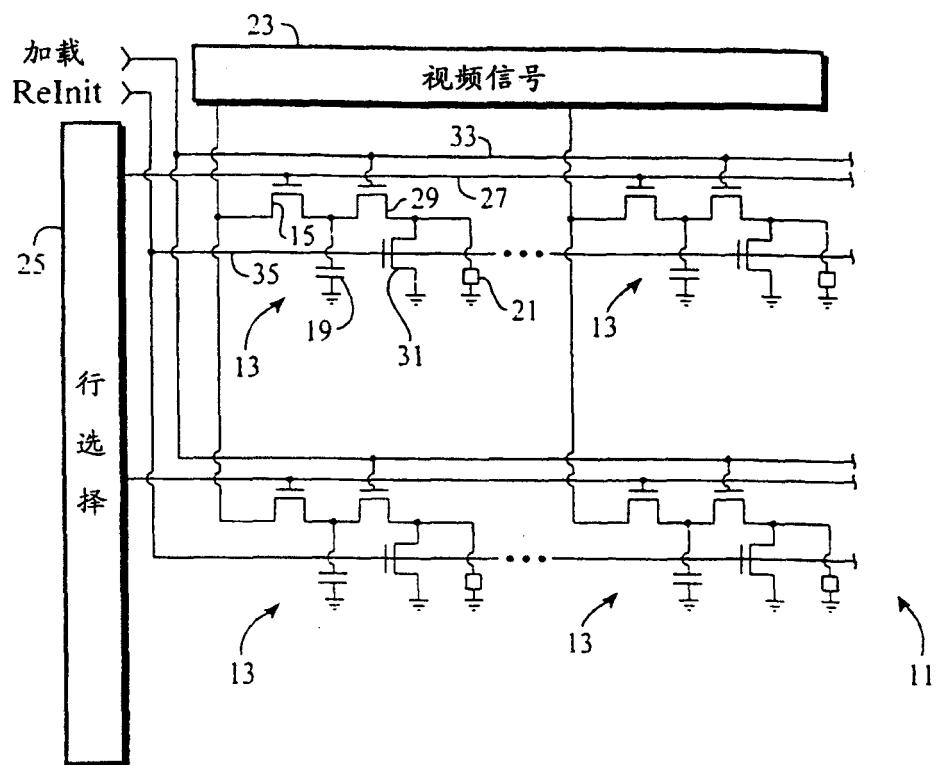
图 3(现有技术)
