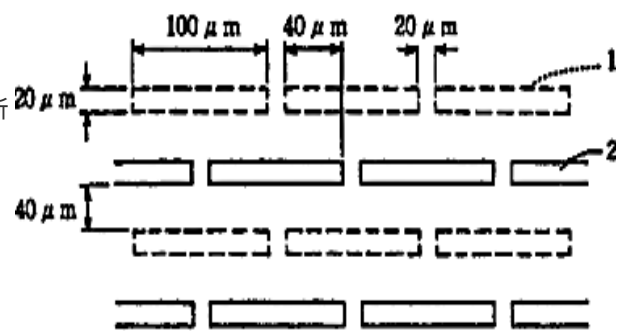
实施例1的狭缝图形
