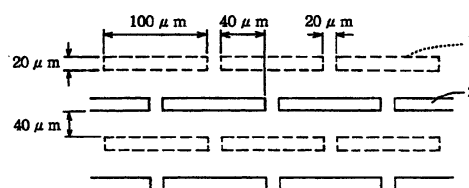
实施例 1 的狭缝图形
