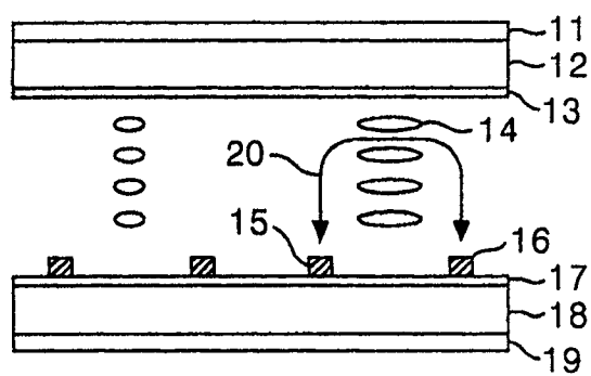
图 1 现有技术
