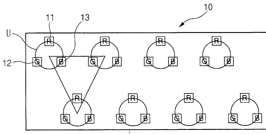
图 2 (现有技术)
