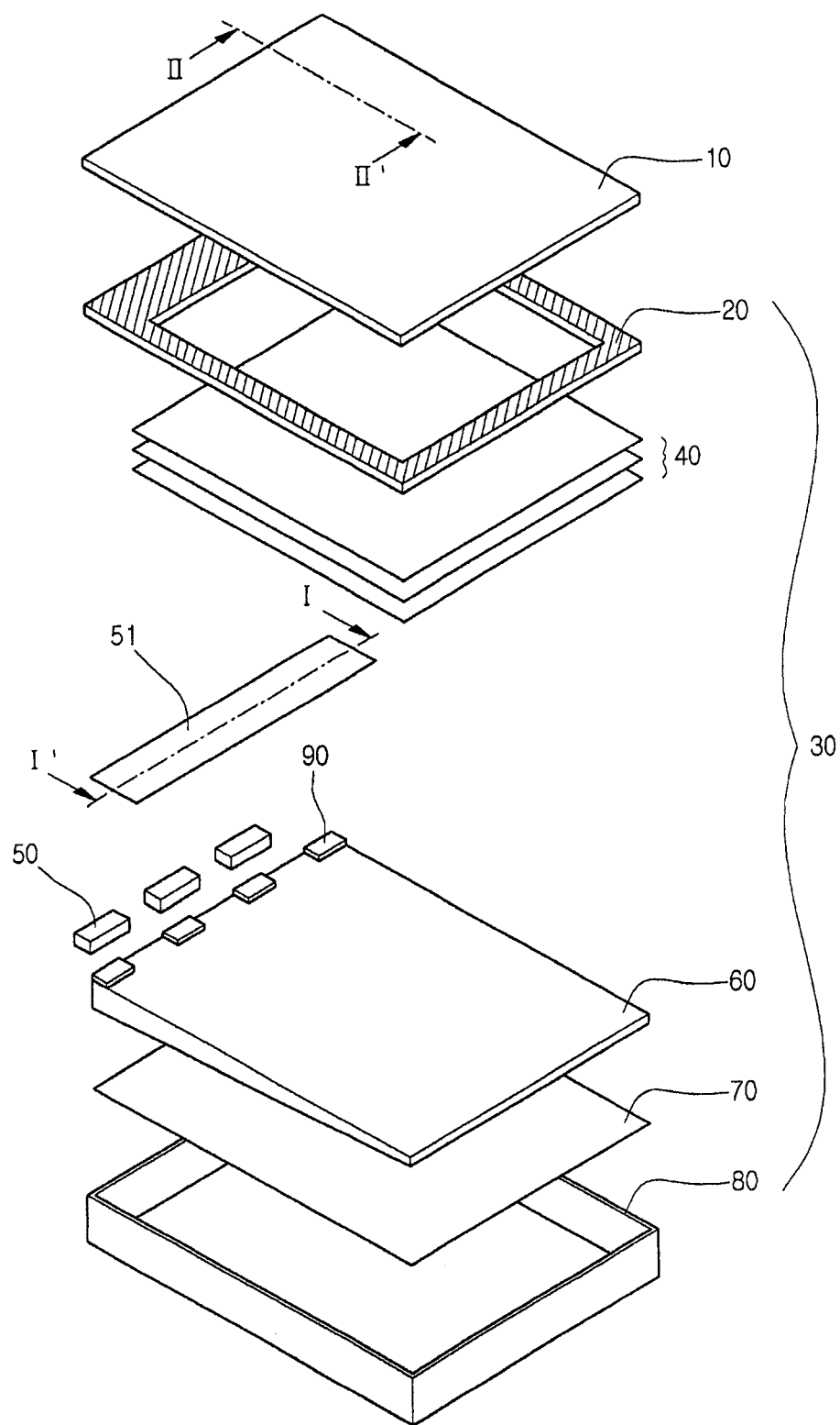
图 1 (现有技术)
