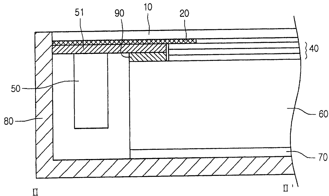
图 3（现有技术）
