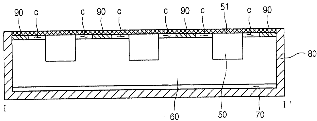
图 2（现有技术）
