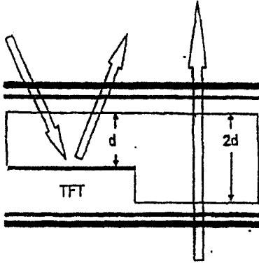
双盒间隙
