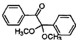
IRGACURE 651
