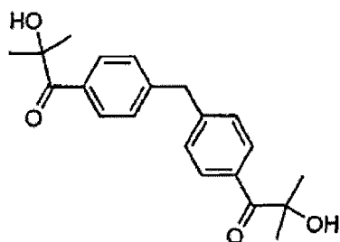
IRGACURE 127
