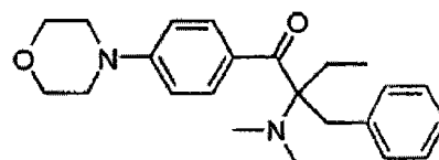
IRGACURE 369
