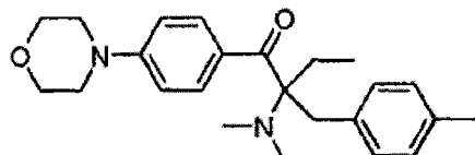
IRGACURE 379
