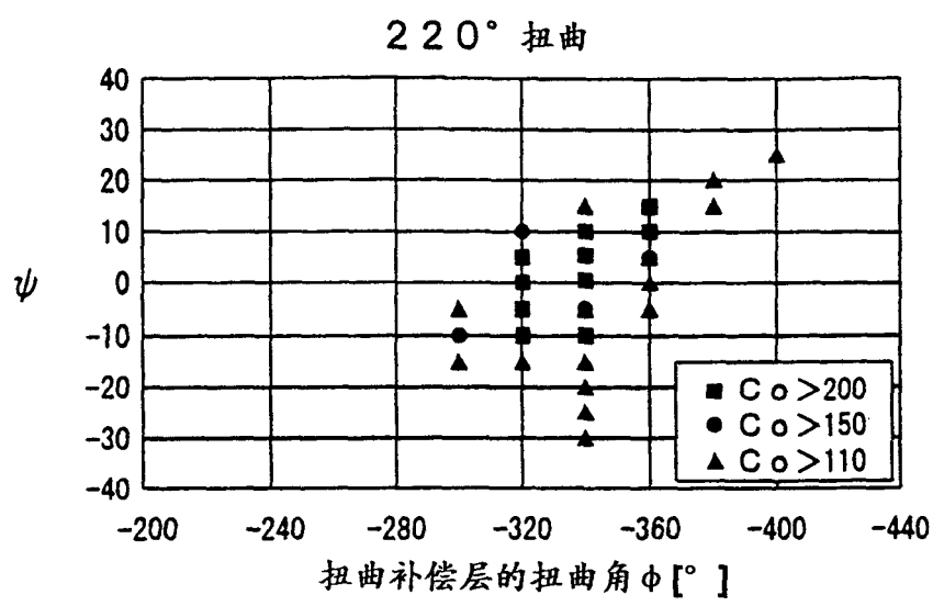
图 12(a) 2 3 0° 扭曲
