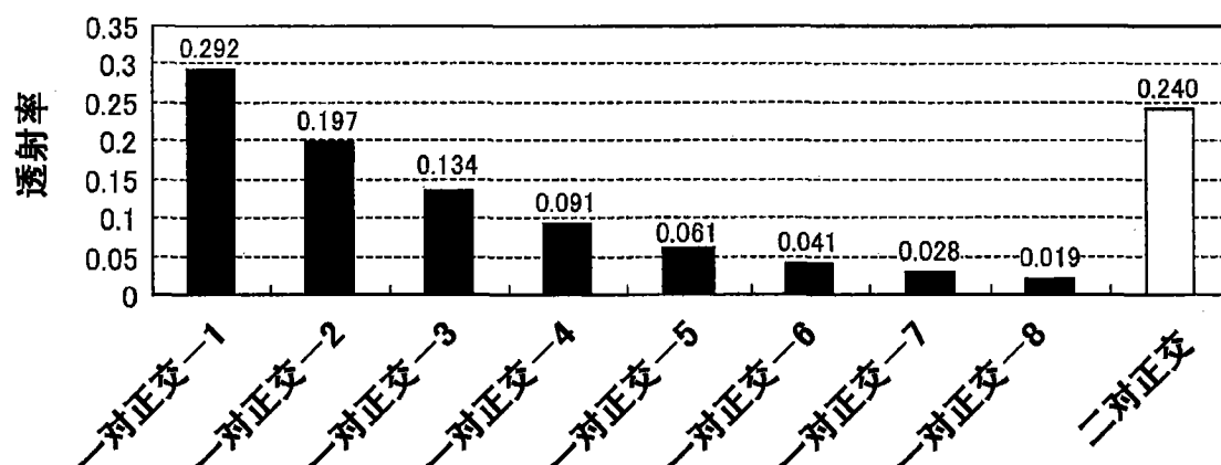
平行透射率(方位角 45^\circ 、极角 60^\circ )
