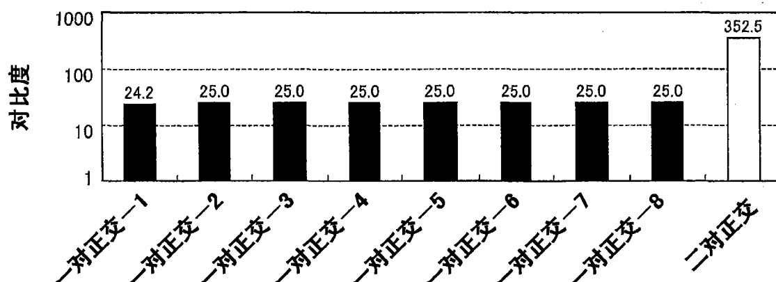
对比度(方位角 45^\circ 、极角 60^\circ )
