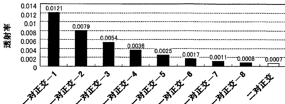
透射率、正交透射率(方位角 45^\circ 、极角 60^\circ )
