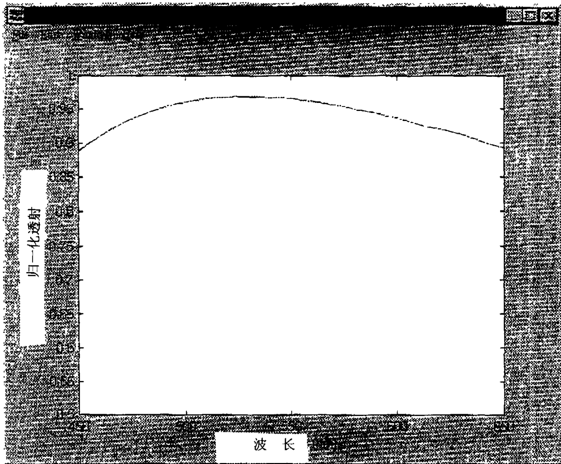
图3 - 140度扭曲亚稳状态的波长-透射曲线图 (40, 40(-50), 95(5), 0.38 构型)
