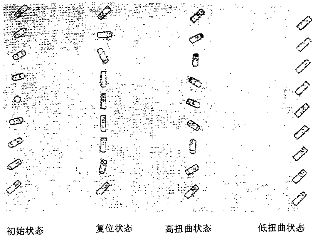
图 1 不同状态下的 LC 指示器的构型
