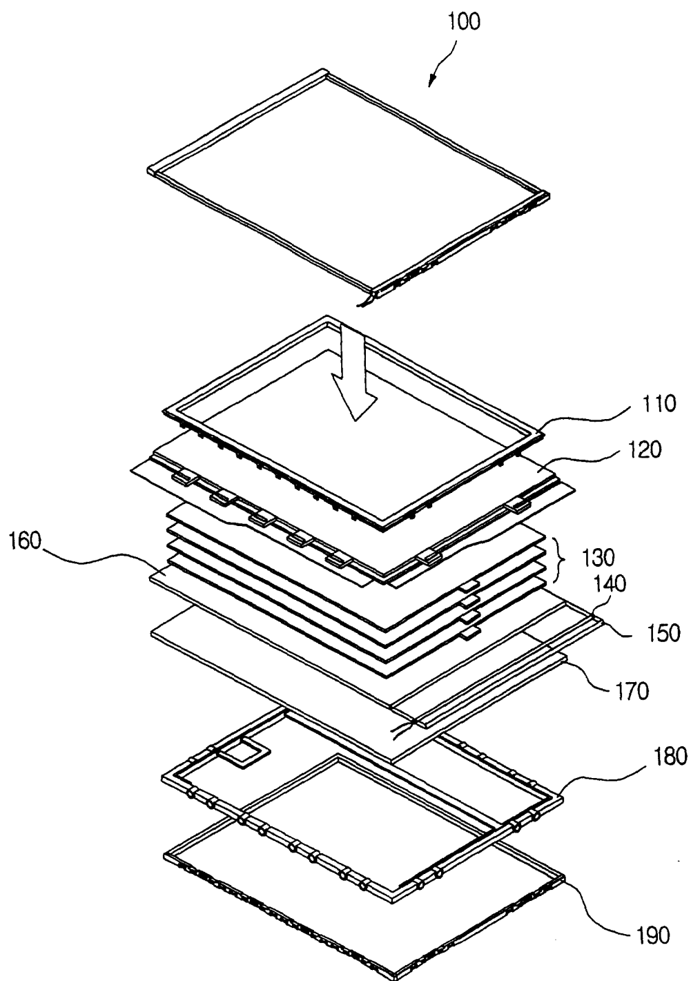
图 1 现有技术
