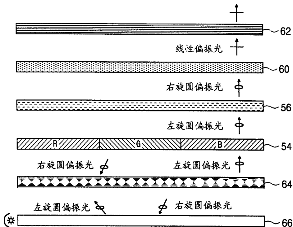
图 2 (背景技术)
