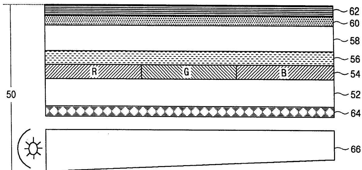
图 2 (背景技术)
