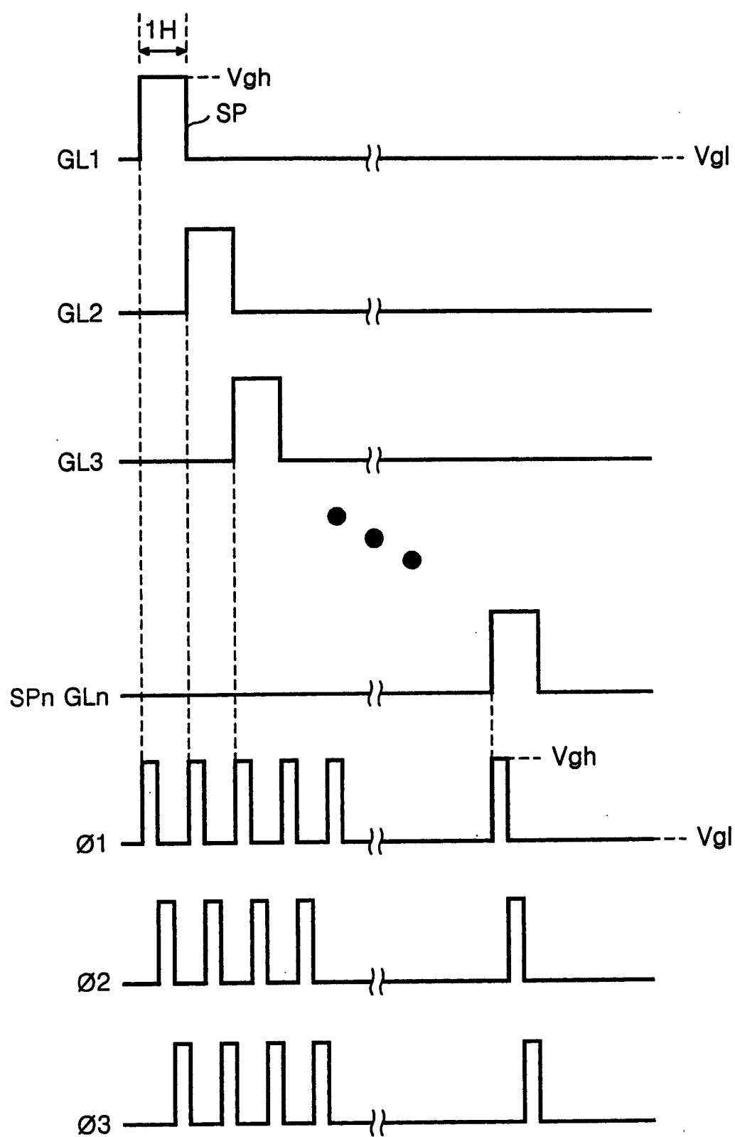
图 2 现有技术
