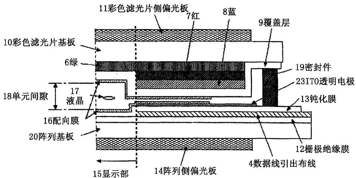
A-A' 剖视图
