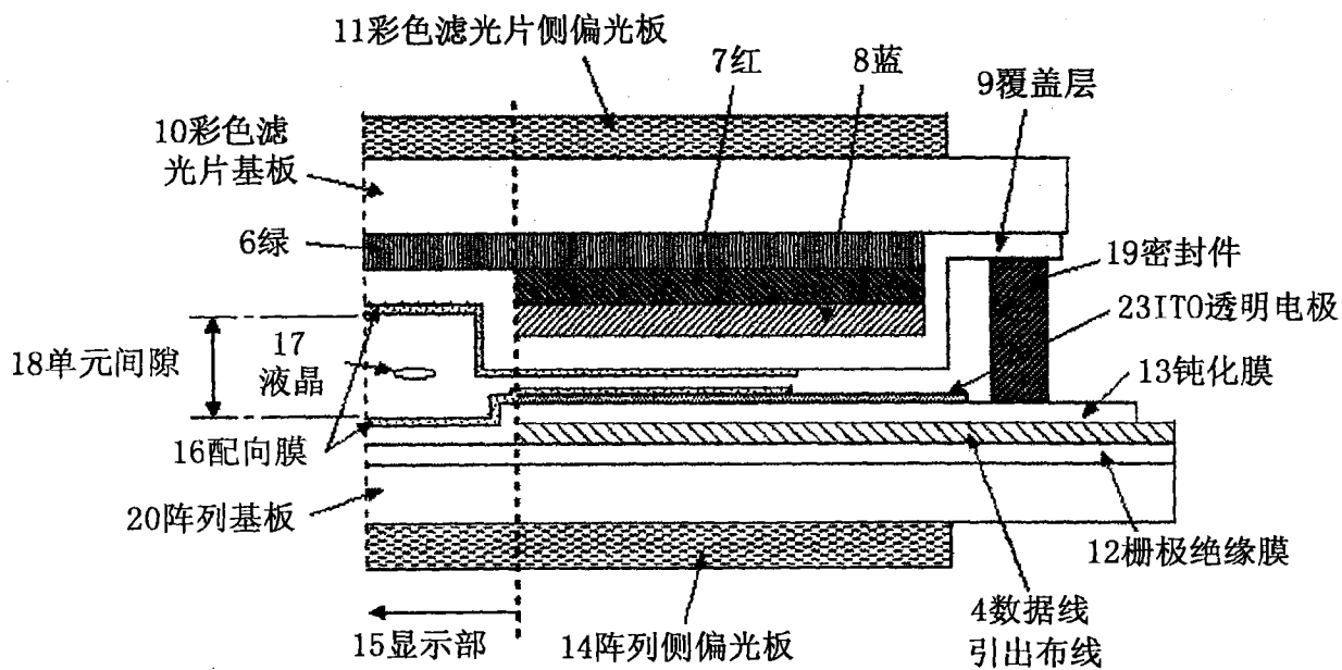
A-A' 剖视图
